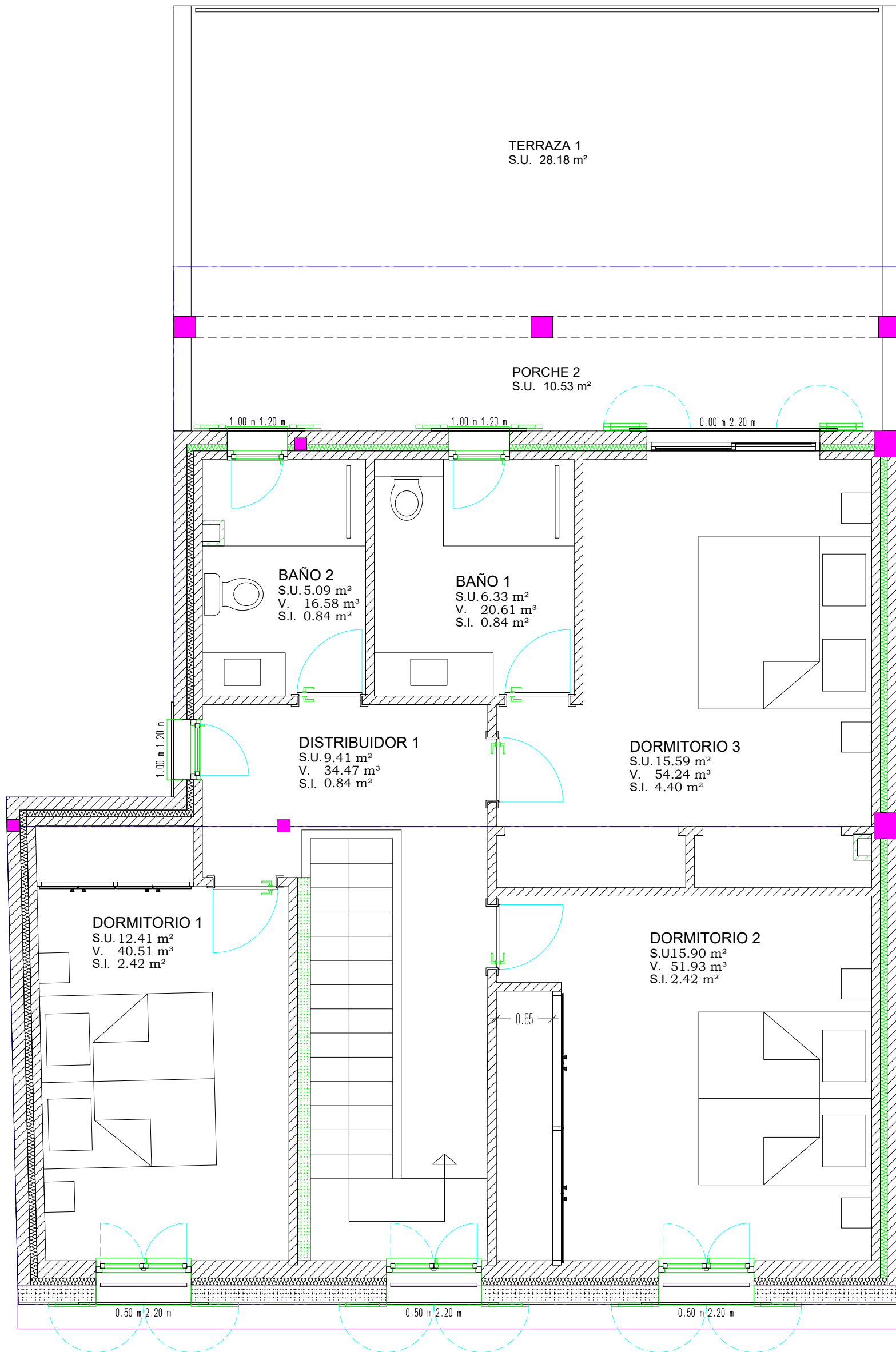
PLANTA PISO E:1/50
